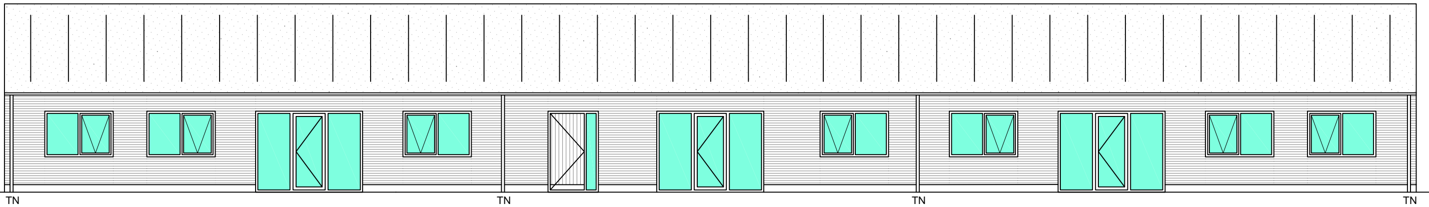
Facade mod nord (Bolig 3, 4 og 5) Facade mod nord (Bolig 6, 7 og 8) Facade mod vest (Bolig 11, 12 og 13)
